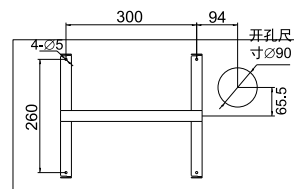
吸顶式支架安装尺寸及开孔尺寸
