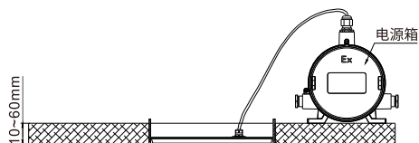
内嵌式安装(Q)
