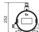
电源箱外形尺寸
