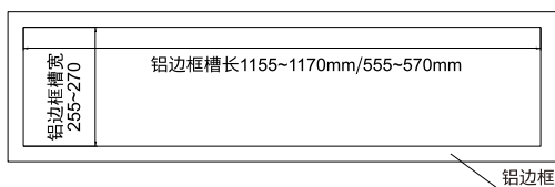
内嵌式安装开槽尺寸
