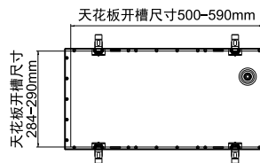
搭扣式安装开槽尺寸
